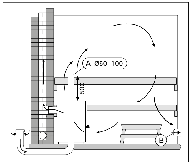
Figure 6. Mechanical exhaust ventilation Abbildung 6. Mechanische Entlüftung
